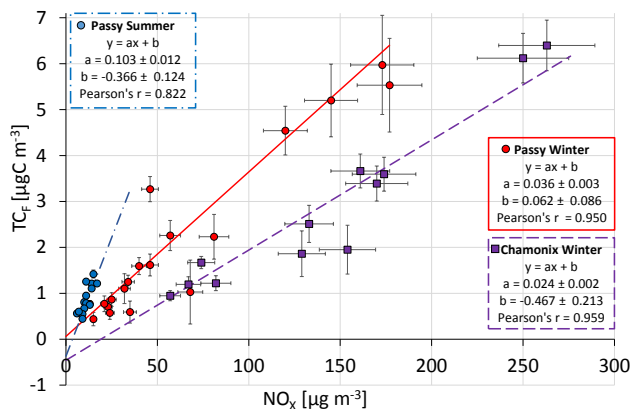
Figure 1 : Comparaison entre les concentrations journalières en carbone fossile (TC F ) et en NO x . Tous les échantillons hivernaux montrent une forte corrélation entre TC F et NO x avec une ordonnée à l'origine proche de zéro, montrant que la majeure partie de TC F provient de la combustion de fuel fossile. Les paramètres des régressions linéaires ont été calculés en prenant en compte les intervalles de confiance sur chaque point (95 %).
