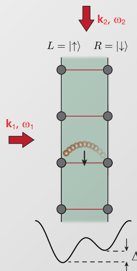
Continuum: I. B. Spielman Nature 471, 83 (2011)
