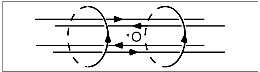
Figure 1 - Un exemple de piège magnétique couramment utilisé (piège de Ioffe-Pritchard). Ce piège est constitué par quatre fils parallèles, parcourus par des courants deux à deux opposés, qui assurent le confinement transverse des atomes. Le confinement longitudinal provient des deux bobines circulaires, parcourues par un même courant. La distance entre ces deux bobines doit être supérieure à leur rayon, pour que le module du champ magnétique présente un minimum en O . Expérimentalement, le champ magnétique en O est de l'ordre de 10^{-4} teslas.
