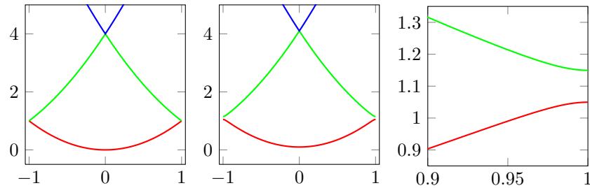
FIGURE 2.7. Bandes d'énergies E_n(q) (unité de E_r ) en fonction de q/k , pour un potentiel V_0 \ll E_r : (a) : V_0 = 0 (même chose qu'à la figure 2.4) ; (b) : V_0 = 0.2 E_r ; (c) : zoom sur le bord de bande q \approx k pour le cas V_0 = 0.2 E_r . On voit qu'un gap de largeur \approx V_0/2 s'ouvre.
