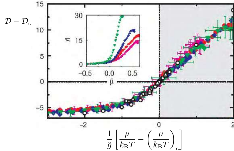
FIGURE 6. Ecart entre la densité dans l'espace des phases \mathcal{D} et sa valeur critique \mathcal{D}_c , en fonction du paramètre "universel" défini en (63). Le paramètre \tilde{g} vaut 0.05 (triangles verts), 0.13 (losanges bleus), 0.19 (cercles rouges) and 0.26 (carrés magenta). L'insert représente la variation de \mathcal{D} en fonction de \mu/k_B T . Ces mesures sont faites sur un gaz de césium au voisinage d'une résonance de Feshbach. Figure extraite de HUNG, ZHANG et al. (2011).
