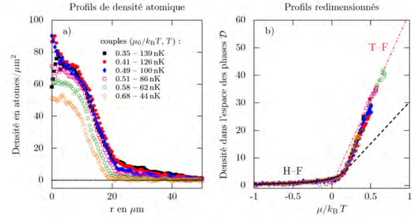
FIGURE 4. Vérification de l'invariance d'échelle pour un gaz 2D de ^{87}\text{Rb} en interaction relativement faible, \tilde{g} = 0.1 . Les profils de densité \rho(r) mesurés dans un potentiel V(r) se regroupent sur une courbe unique si on trace la densité dans l'espace des phases \mathcal{D}(r) = \rho(r)\lambda_T^2 en fonction de \mu_{\text{loc}}(r)/k_B T . Les deux régimes Hartree-Fock (HF) et Thomas-Fermi (TF) correspondent respectivement au cas faiblement et fortement dégénérés. Figure extraite de la thèse de Tarik YEFSAH (2011).
