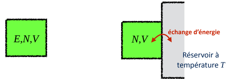
FIGURE 1. Gauche, ensemble micro-canonique : système isolé décrit par trois variables extensives : l'énergie E , le nombre de particules N et le volume V . Droite, ensemble canonique : système pouvant échanger de l'énergie avec un réservoir qui impose ainsi sa température T (variable intensive). Le volume et le nombre de particules du système restent fixés.
