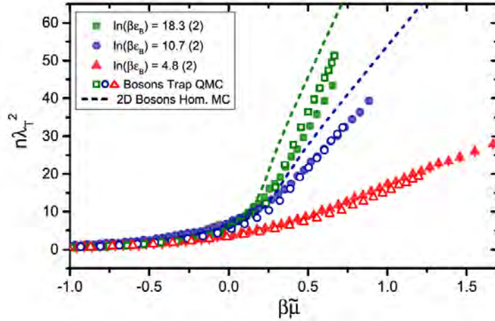
FIGURE 5. Symboles fermés : équations d'état mesurées pour un gaz de molécules ^6\text{Li}_2 avec un paramètre d'interaction \tilde{g} = 0.60 (carrés), 1.07 (cercles), 2.75 (triangles). Les lignes pointillées donnent la prédiction obtenue par simulation de champ classique (PROKOF'EV & SVISTUNOV 2002). Les symboles ouverts donnent le résultat d'une simulation de Monte Carlo quantique. Figure extraite de BOETTCHER, BAYHA et al. (2016).
