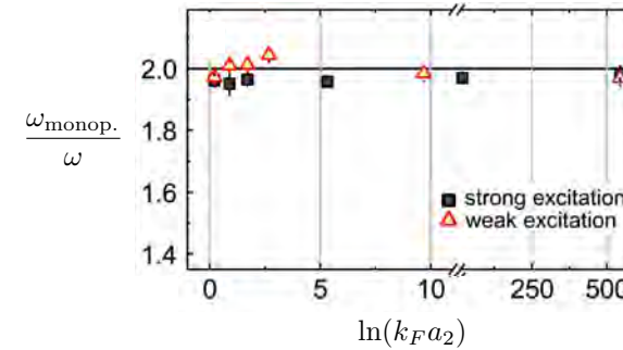
FIGURE 9. Fréquence du mode monopolaire d'un gaz 2D de fermions ( ^{40}\text{K} ) au voisinage d'une résonance de Feshbach. La longueur de diffusion a_2 est mesurée ici en unités du vecteur d'onde de Fermi k_F ( E_F = \hbar^2 k_F^2 / 2m \approx 5 à 8 \text{ kHz} \times \hbar ). On trouve que la fréquence du mode monopolaire reste très proche de la valeur prédite dans le cadre de l'invariance d'échelle, même quand la longueur de diffusion a_2 devient grande. Figure extraite de VOGT, FELD et al. (2012).
