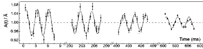
FIGURE 8. Oscillation temporelle de l'aire transverse d'un gaz 3D de rubidium confiné dans un piège « cigare ». L'oscillation se fait à une fréquence égale (à la précision de mesure près) au double de la fréquence transverse du piège. Ce mode d'oscillation n'est que très faiblement amorti (facteur de qualité > 2000 ). Figure extraite de CHEVY, BRETIN et al. (2001).
