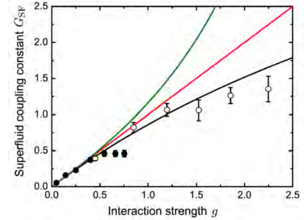
FIGURE 7. Paramètre G = m/(\hbar^2 \kappa) , caractérisant le lien entre densité \rho et potentiel chimique \mu à très basse température pour un gaz 2D d'atomes de césium. La théorie de champ classique prédit G = \tilde{g} (ligne droite rouge). La ligne noire continue représente une prédiction basée sur la théorie de Ginzburg–Landau (SACHDEV & DEMLER 2004). Les symboles ouverts ont été obtenus pour un gaz évoluant dans un réseau optique opérant dans un régime où son effet est essentiellement une renormalisation de la masse et de la force des interactions. Figure extraite de HA, HUNG et al. (2013).
