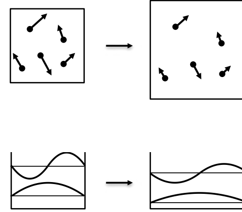
FIGURE 3. Dilatation des longueurs par un facteur \lambda dans le cas classique (en haut) et quantique (en bas).
