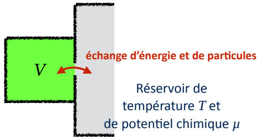
FIGURE 2. Ensemble grand-canonique : le système peut échanger de l'énergie et des particules avec un réservoir, qui impose sa température T et son potentiel chimique \mu (variables intensives). Le volume du système reste fixé.
