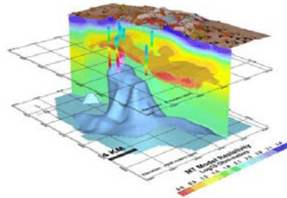
Imagerie 3D Résistivité
