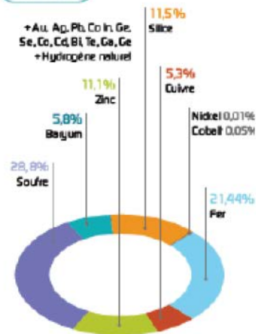
Sulfures hydrothermaux
